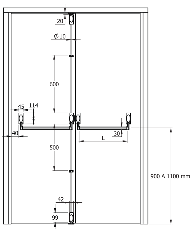
BARRA ANTIPÂNICO NEO DUPLA
