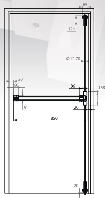
BARRA ANTIPÂNICO TOUCH VERTICAL
