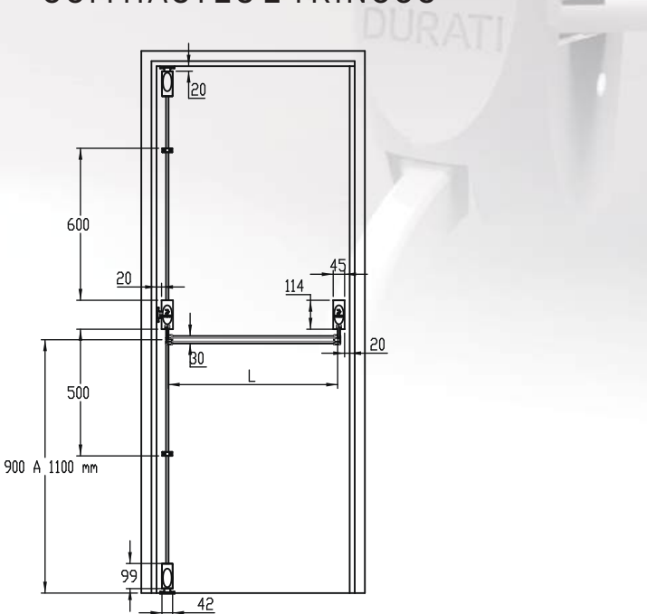
COM HASTES E TRINCOS
