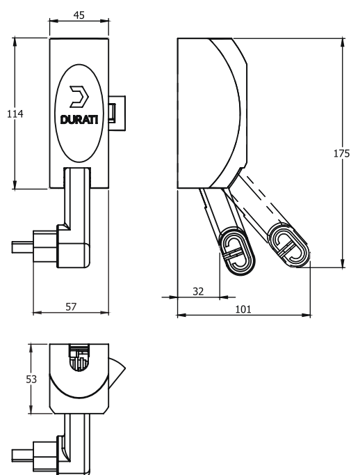
SUORTE P/ BARRA ANTIPÂNICO
