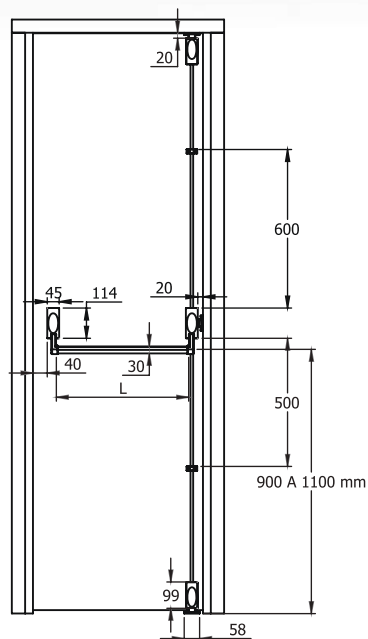
BARRA ANTIPÂNICO NEO SIMPLES COM HASTES E TRINCOS
